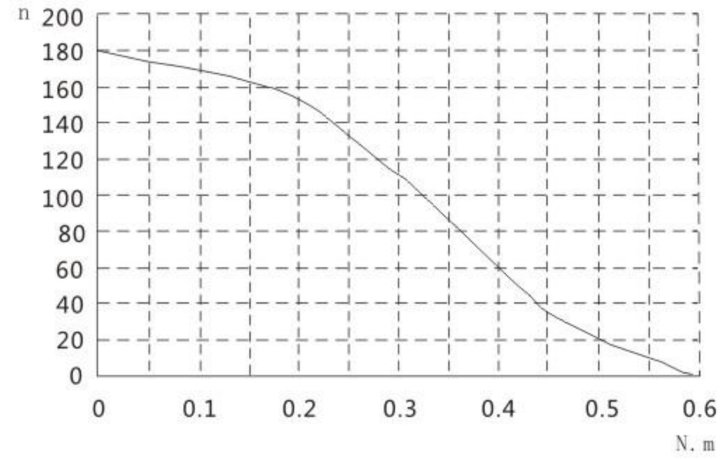
转速-转矩曲线图 Rotation rate-torque cure diagram
